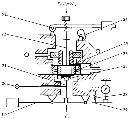
图2 仪器原理图
