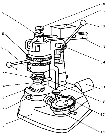
图1 仪器外形图
