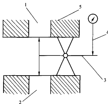
图 3 加荷力检定装置安装示意图
